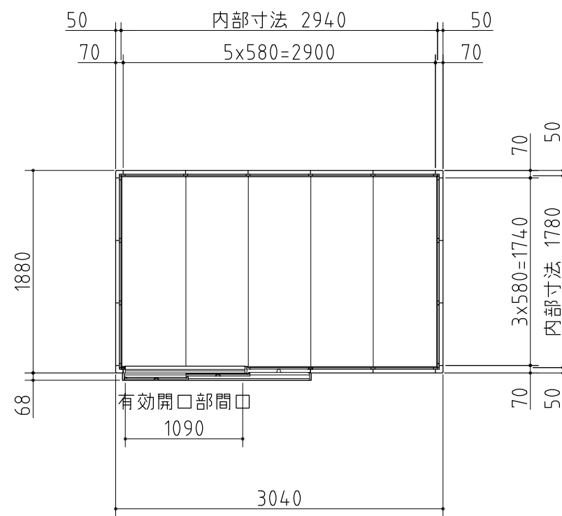
平面図
