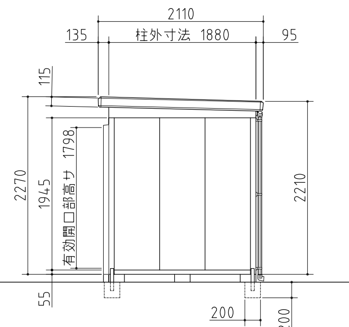
右側面図
