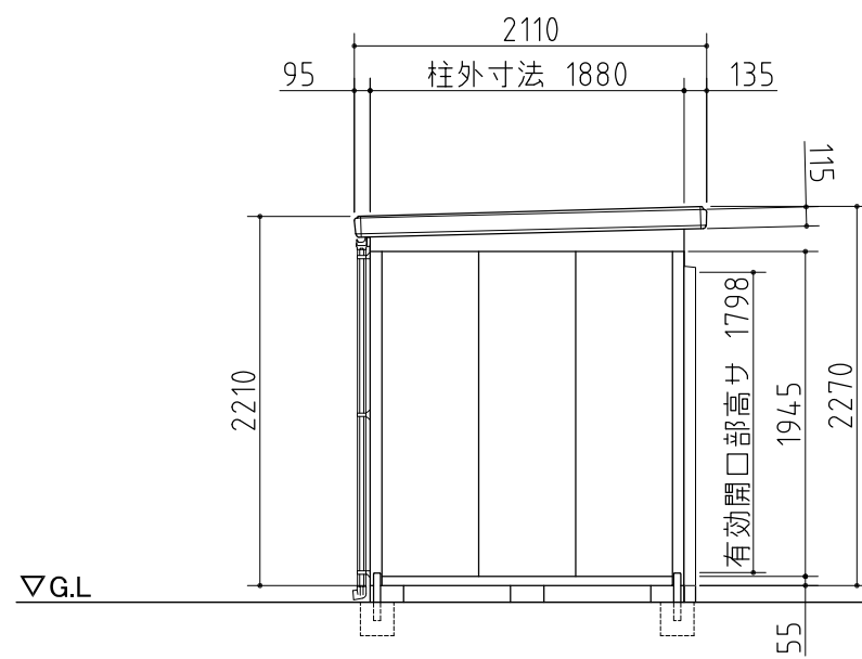
左側面図
